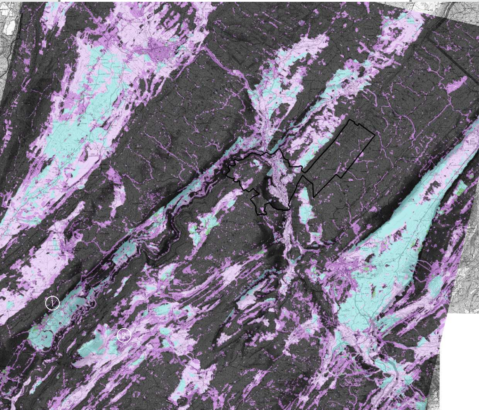
Figure 3.9. Carte des volumes du paysage sur le secteur de Morez (fond : scan25, IGN).
